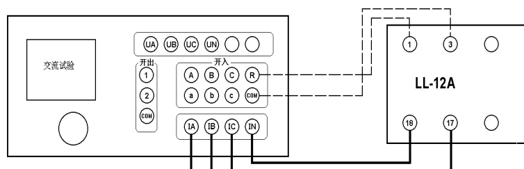
(请尽量采用粗、短接线，或取下继电器就近接线) LL-12A 过电流继电器的接线图
