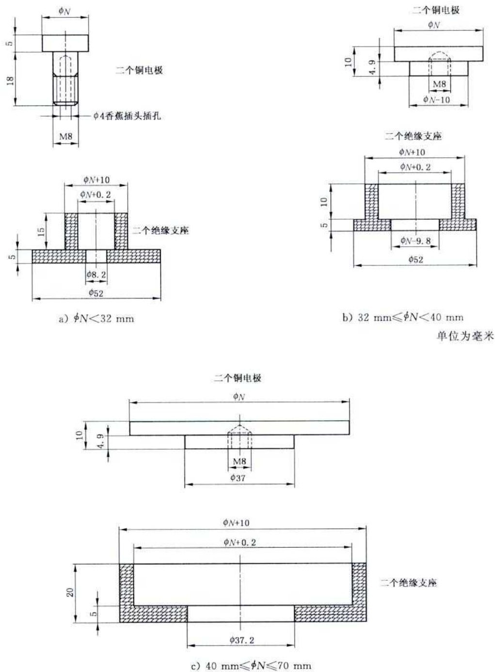
图 A.5 按试品直径配备的保证电极部件结构图
